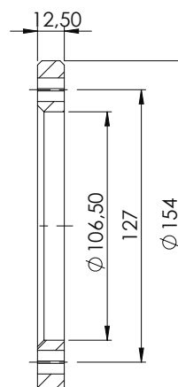
SEÇÃO A-A
